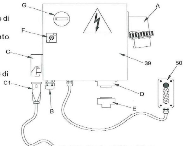
Fig.5-01 Quadro elettrico di base
